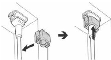
držač priključka mrežnog kabela (isporučen)
