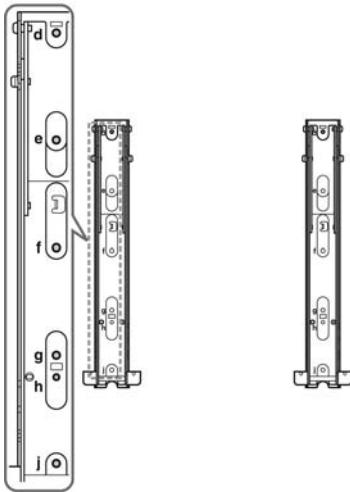
Položaj vijka
